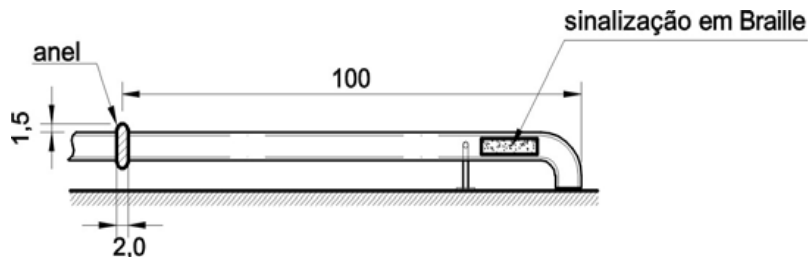
Figura 57 – Sinalização de corrimãos
